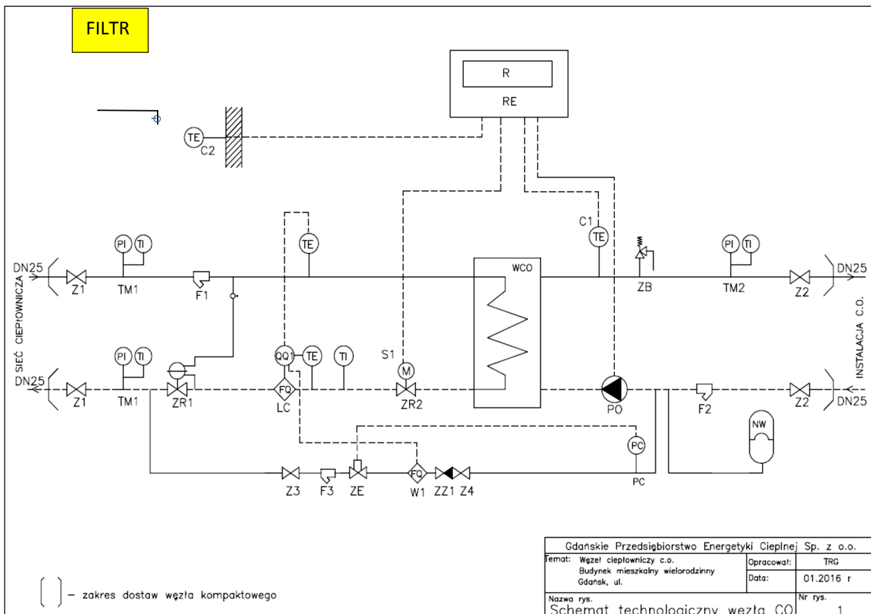
Załącznik nr 9 Schemat technologiczny węzła do 90 kW c.o
