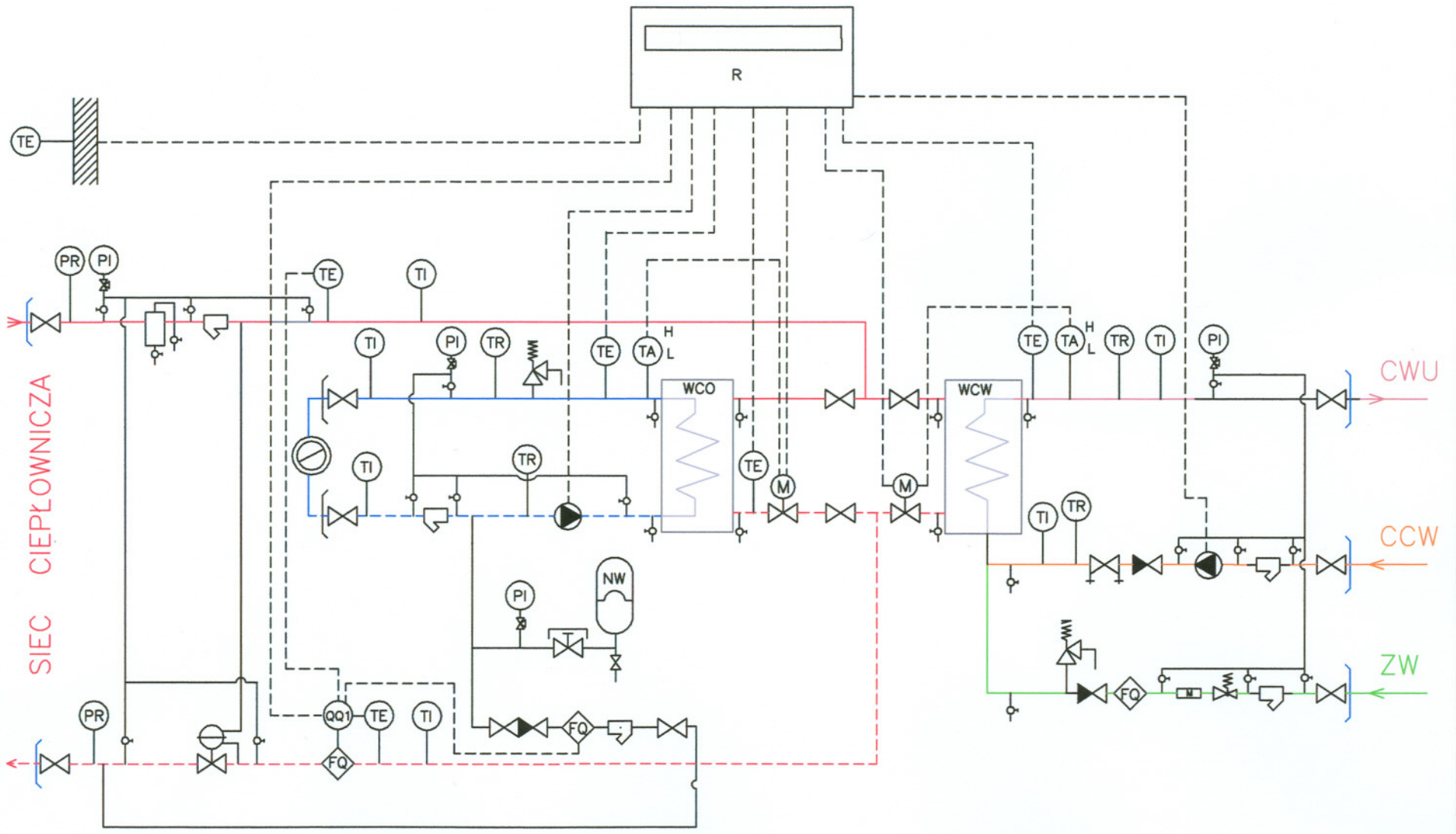
SCHEMAT TECHNOLOGICZNY DWUFUNKCYJNEGO WĘZŁA CO/CWU
