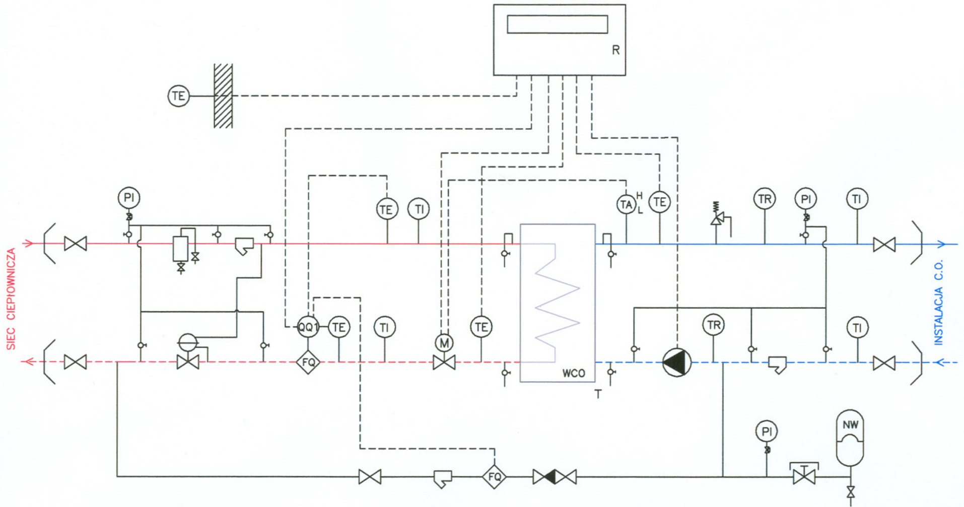
SCHEMAT TECHNOLOGICZNY JEDNOFUNKCYJNEGO WĘZŁA C.O.
